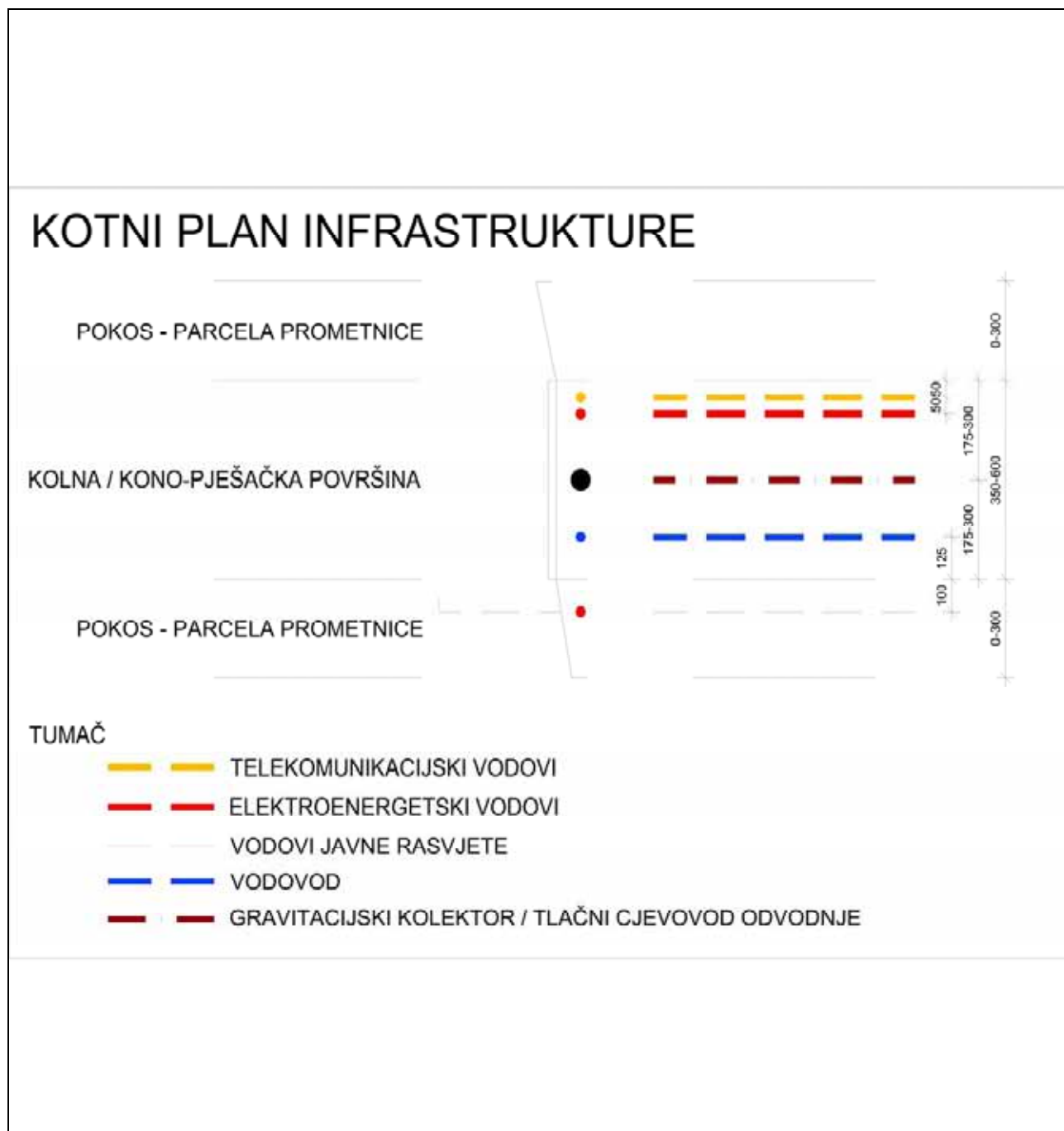
Slika 3-4.: Kotni plan infrastrukture.
