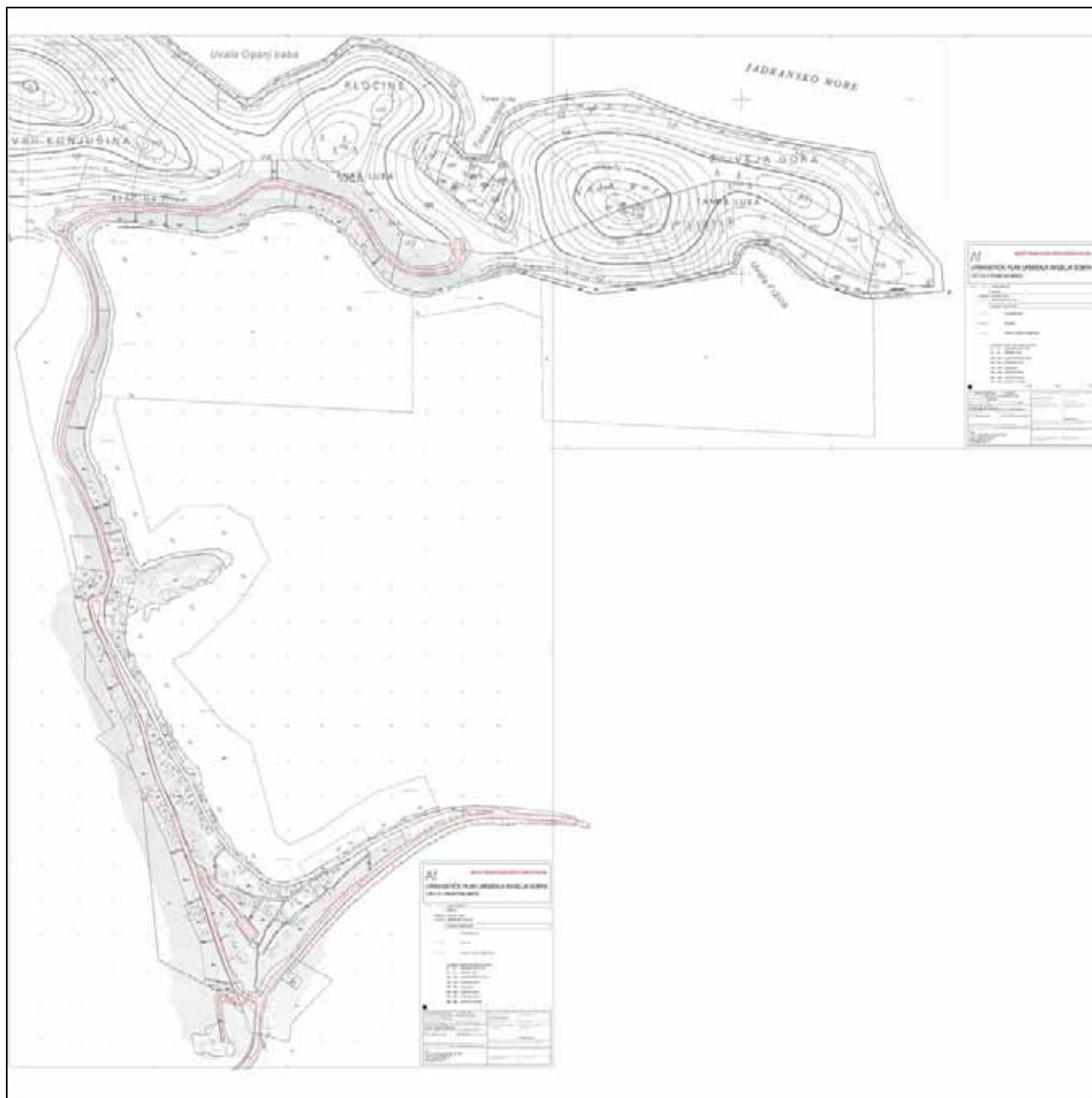
Slika 3-1: Prikaz prometne mreže naselja Sobra. Kartografski prikaz list broj: 2A : „Prometna mreža“ u mjerilu 1:1000.
